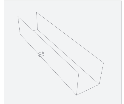
Abbildung 16: Isometrie des Modellraums mit Verbauelement durch einen gegenüber des Fensters befindlichen Gebäuderiegele
